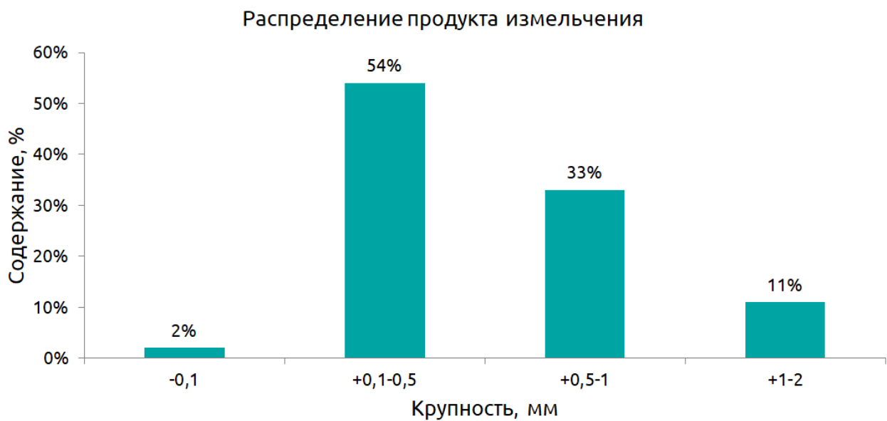
Рис. 6. Распределение продукта измельчения
